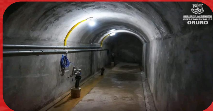
GALERIA DE INSTRUMENTACION PARA MONITOREO DE LA PRESA
